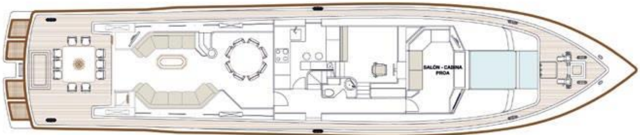
cubierta principal / main deck
