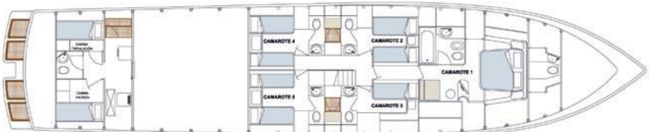
cubierta inferior / lower deck
